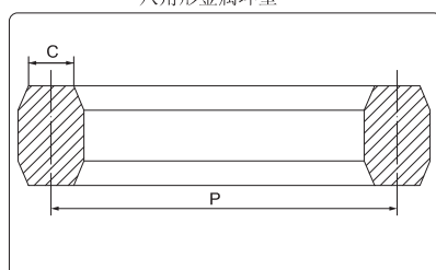
八角形金属环垫
